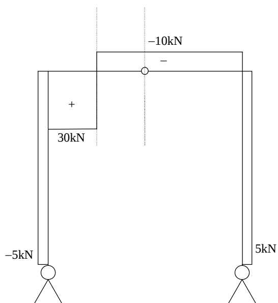
SFD , V
