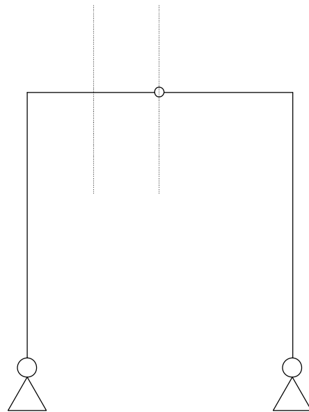
BMD , M
